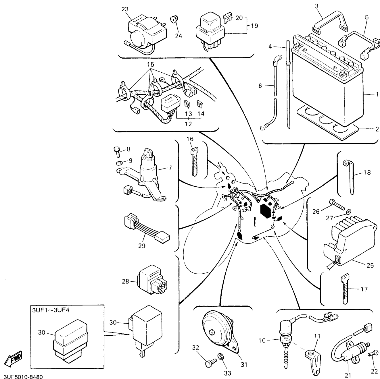
FIG. 48 エレクトリカル 2
