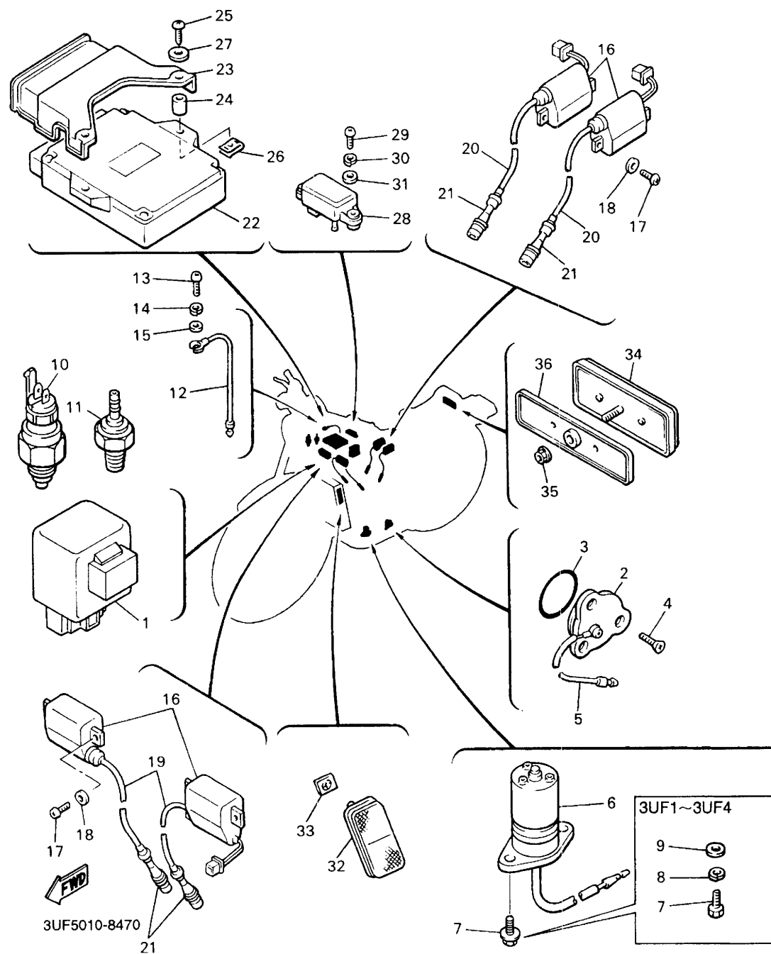
FIG. 47 エレクトリカル 1
