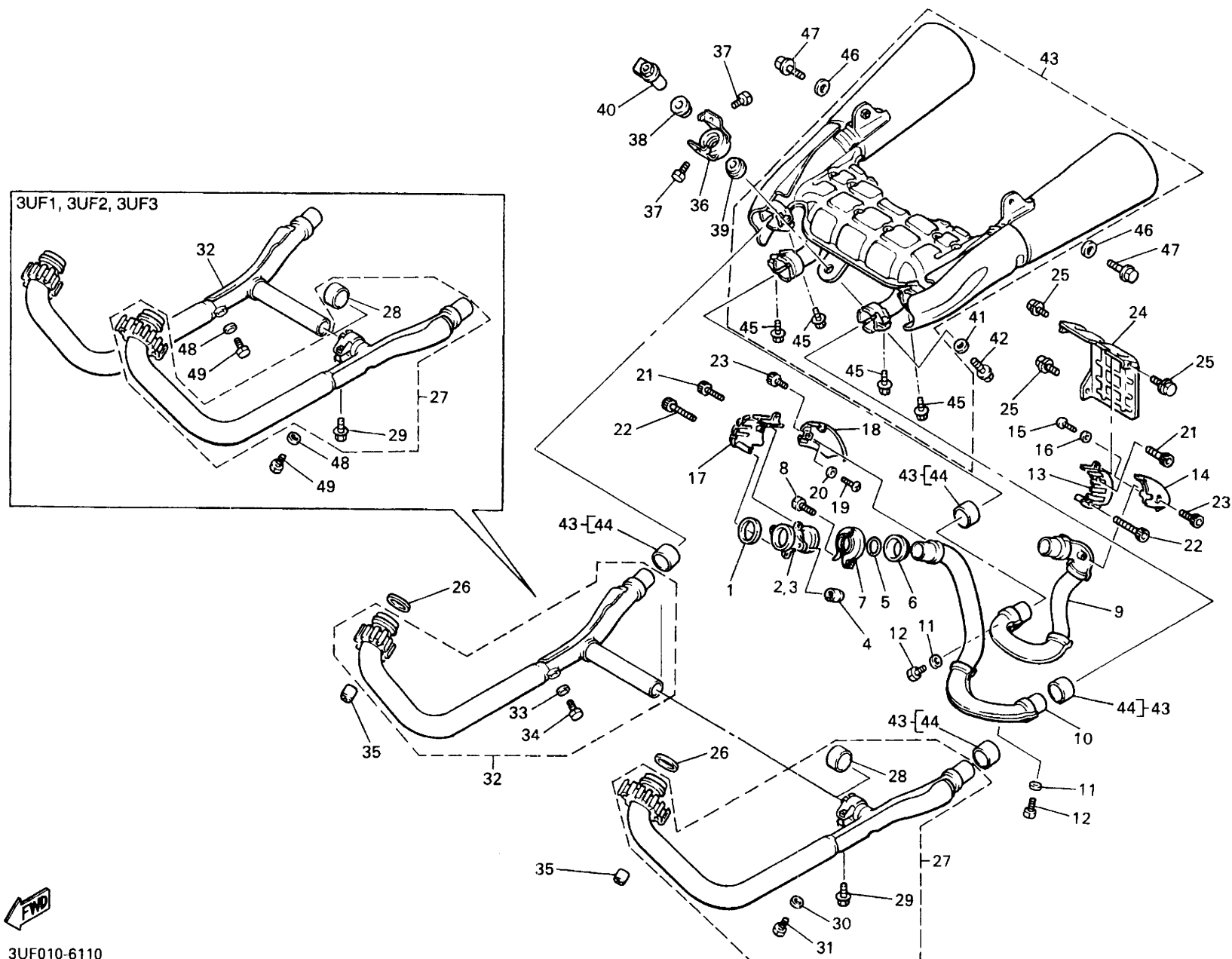
FIG. 11 エキゾースト
