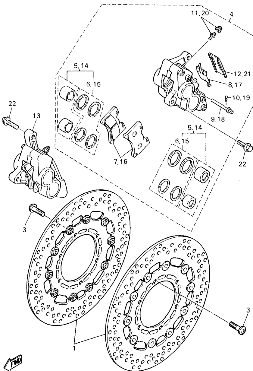
FIG. 32 フロントブレーキキヤリパ
