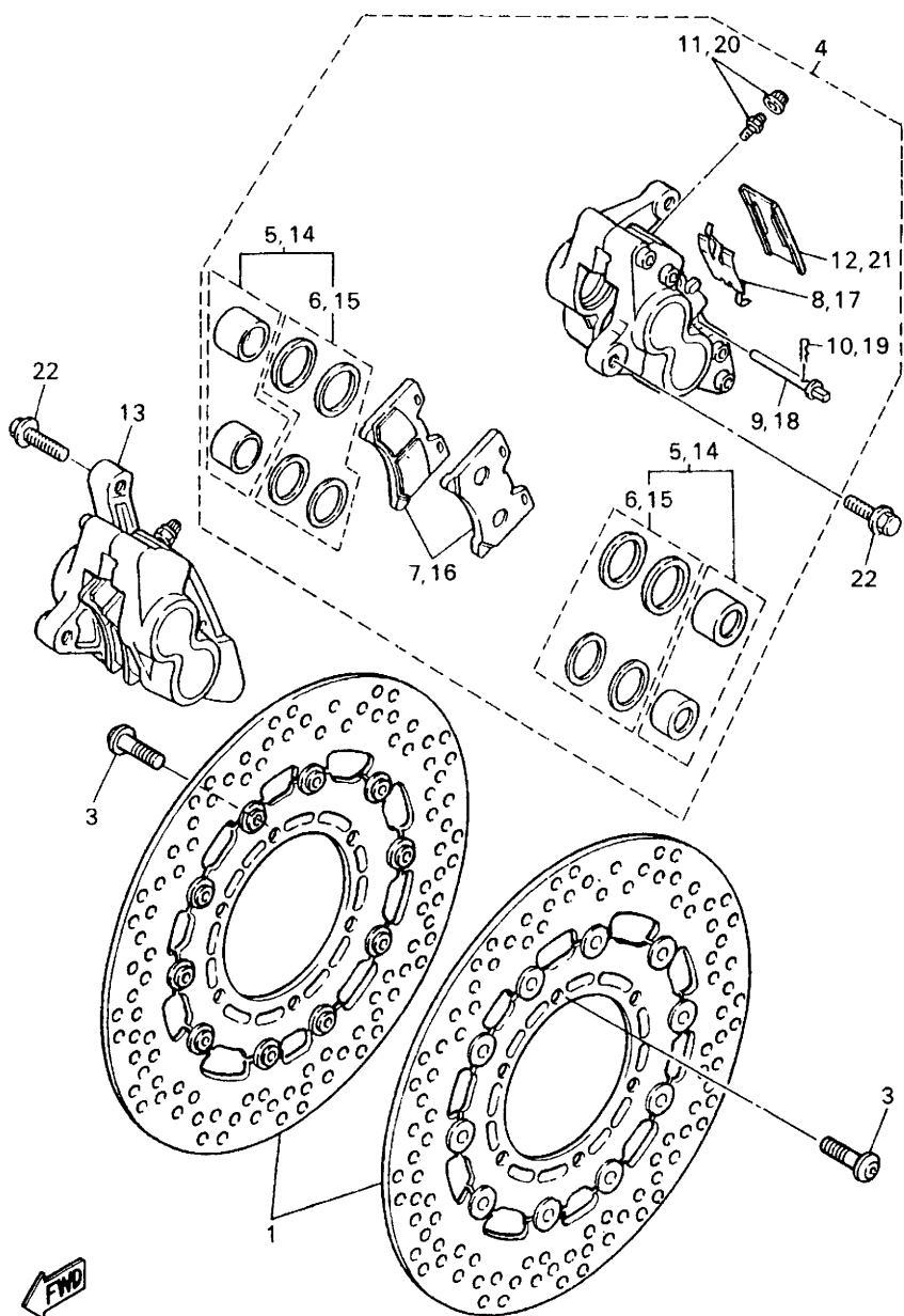
FIG. 32 フロントブレーキキャリパ
