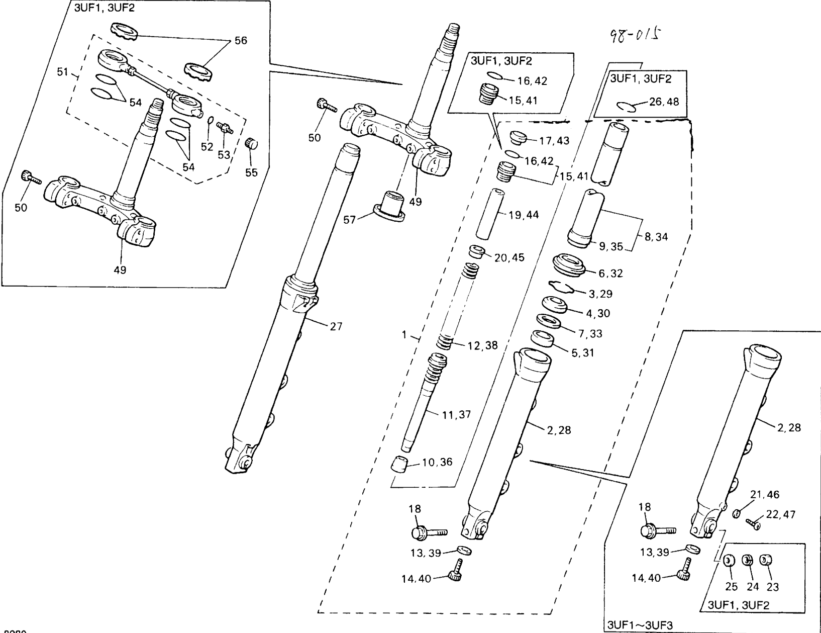
FIG. 28 フロントフォーク
