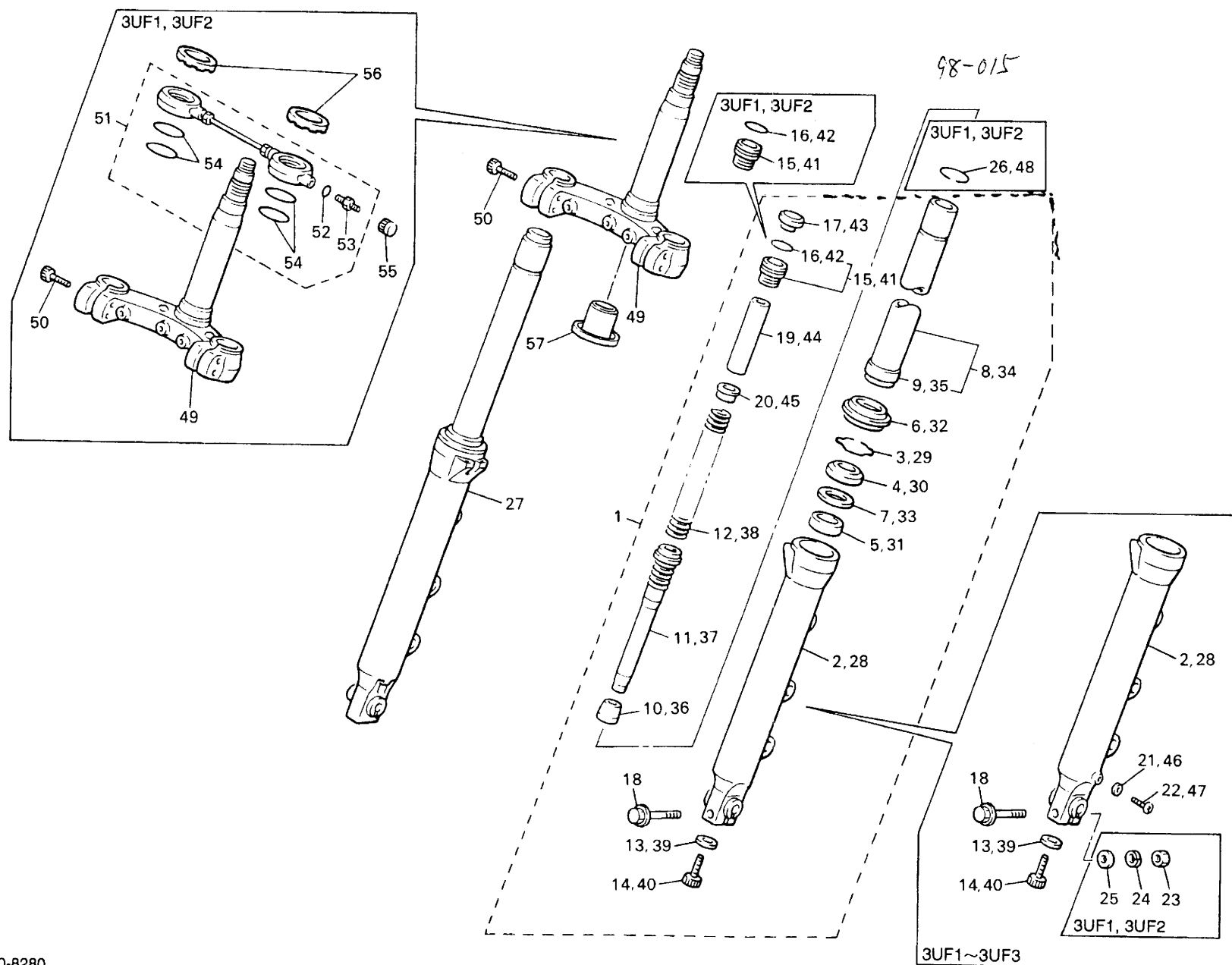
FIG. 28 フロントフォーク
